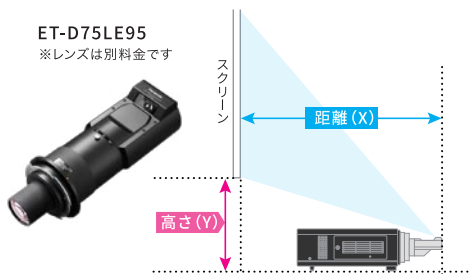
ET-D75LE95装着時 投影距離(16:10) 単位:m
